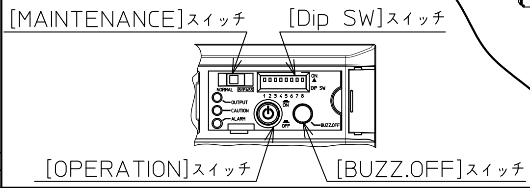
操作部詳細図 (表示部カバーを開けた状態)
