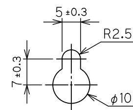
A部詳細
