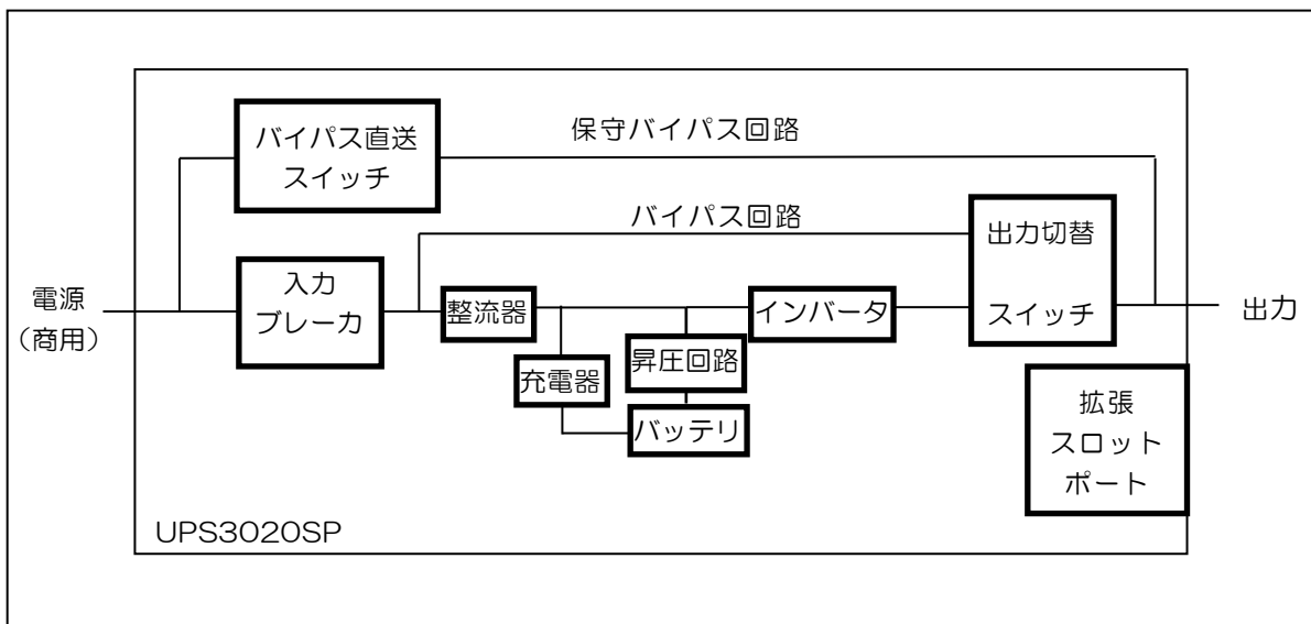
UPS3020SP 概略構成図
