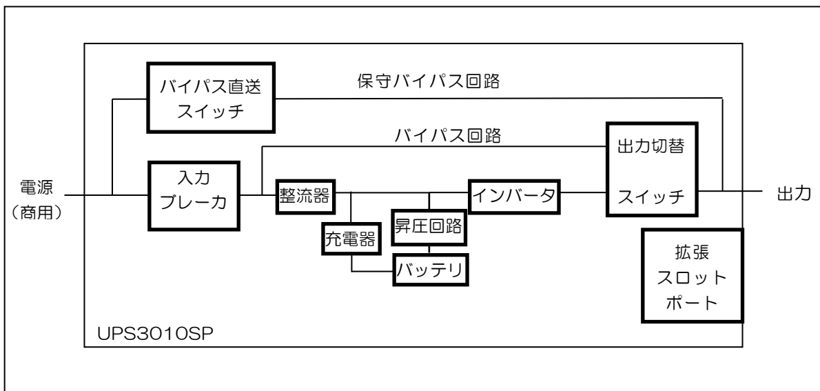
UPS3010SP 概略構成図
