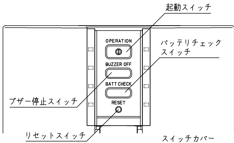
スイッチカバー内部
