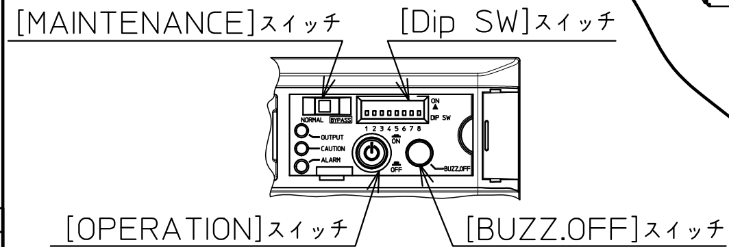
操作部詳細図 (表示部カバーを開けた状態)
