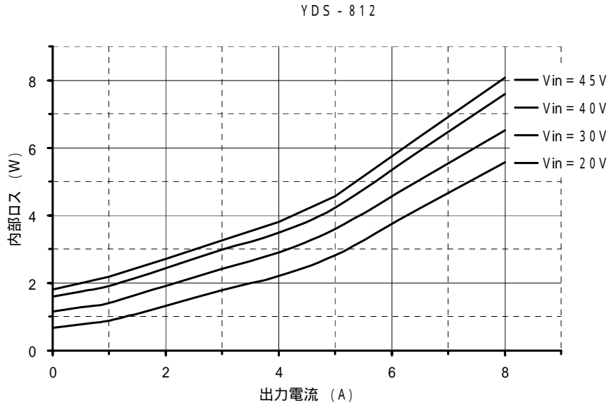
図6. 内部ロス曲線 (Ta=25 代表例)
