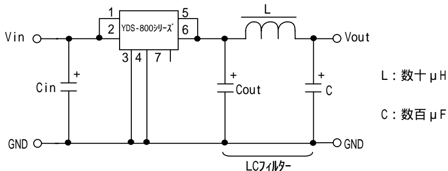
図25. 低ノイズ化
