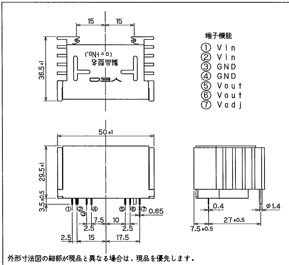
図1. 外形寸法図
