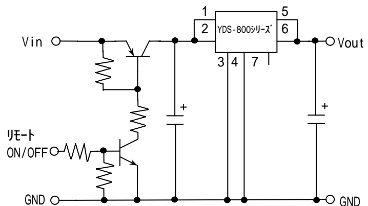
図28. リモートON/OFF
