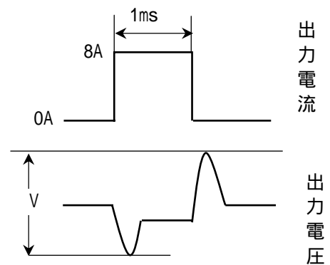
図21. 出力波形
