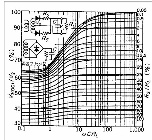
図15. O.H.Schade のグラフ
