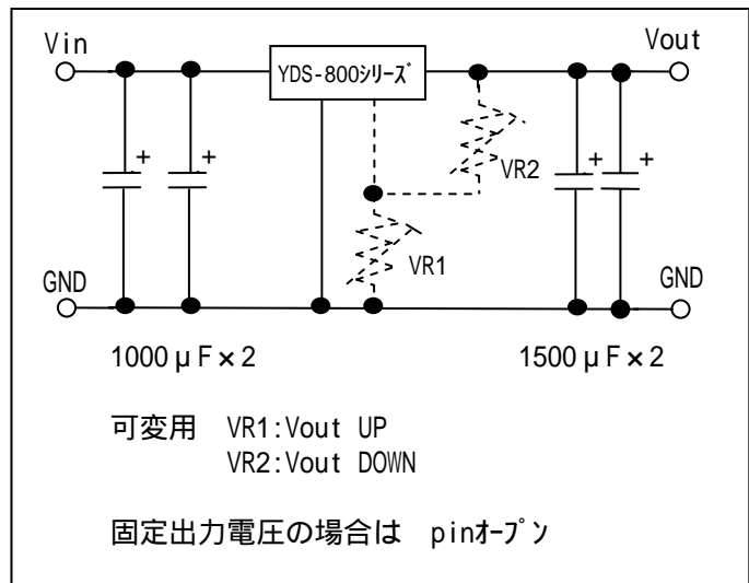
図10. 外部接続図
