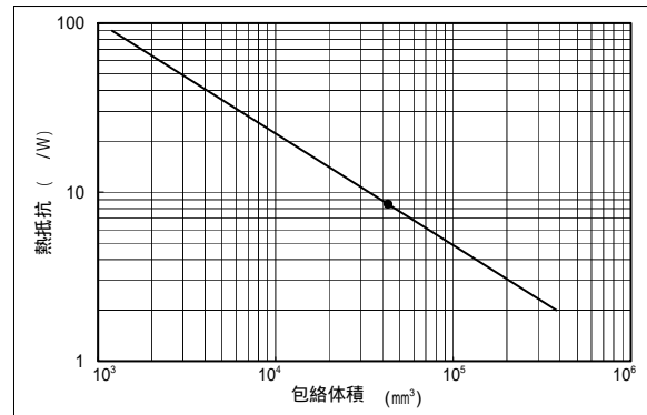
図9. 放熱フィンの包絡体積と熱抵抗
