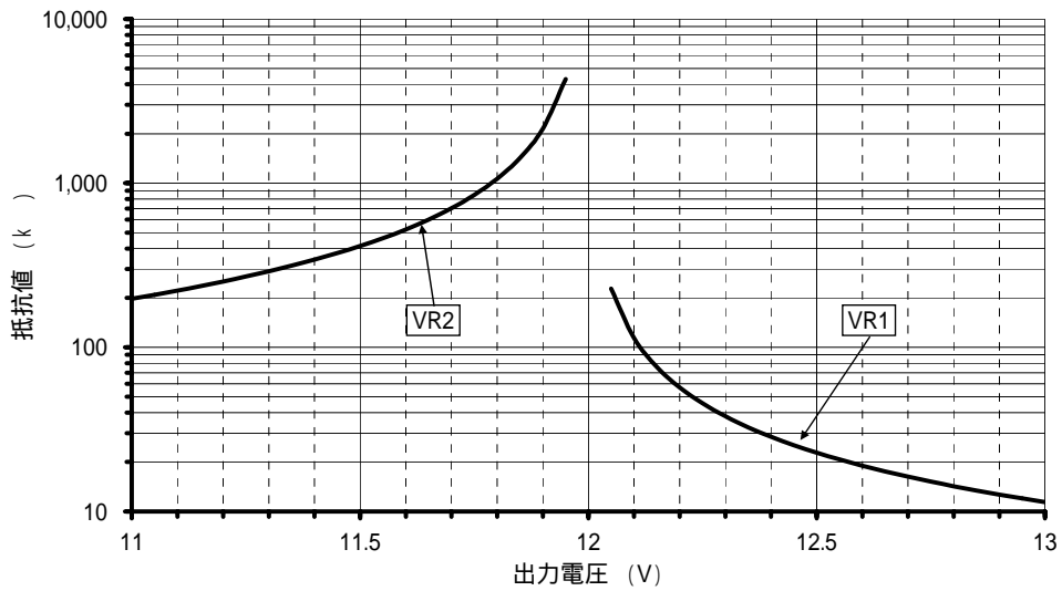
図11. 出力電圧可変抵抗のグラフ
