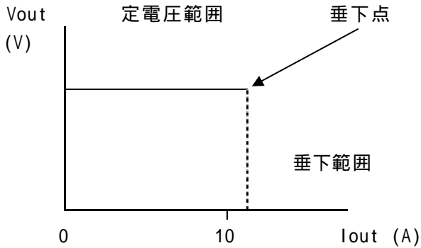
図22. 過電流垂下特性
