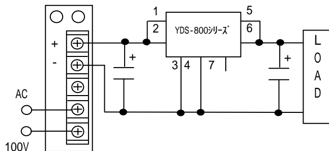
図12. 標準電源、バッテリーで使用する場合
