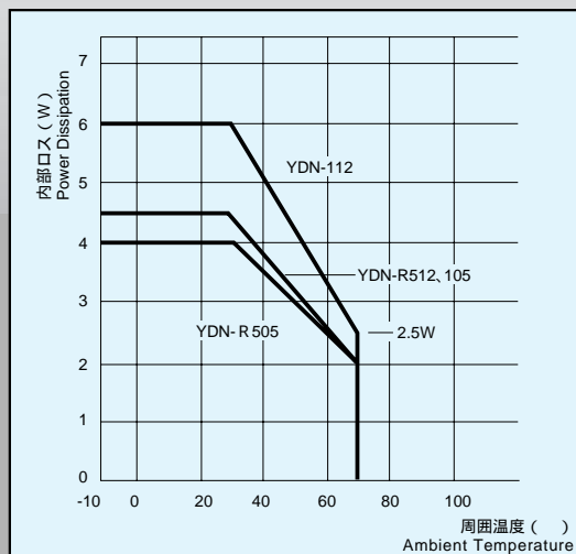
減定格曲線
