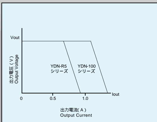
出力電圧垂下曲線 Output Characteristics of Current Limiter
