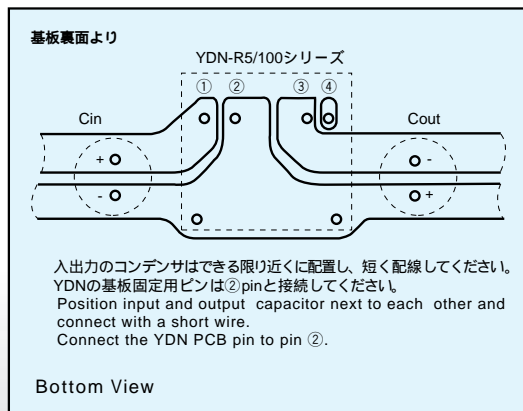
参考パターン図 Recommended Set-UP
